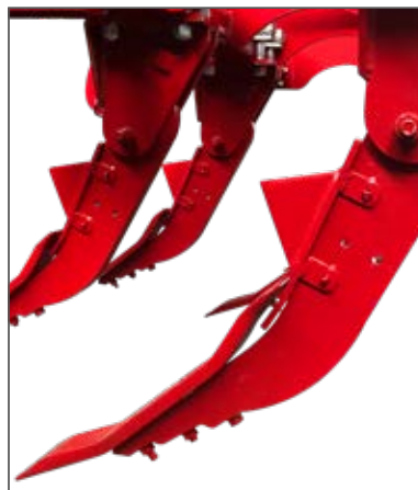
Espulsore con zappette Ejector with hoes
